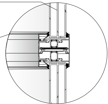
Dreifachscheibe
