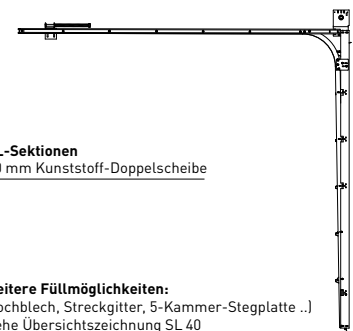
Normal-Beschlag
